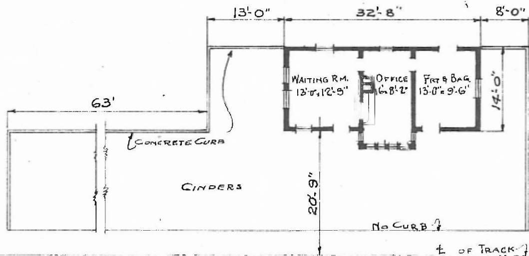
FLOOR PLAN SCALE: \frac{1}{8}'' = 1'-0''
