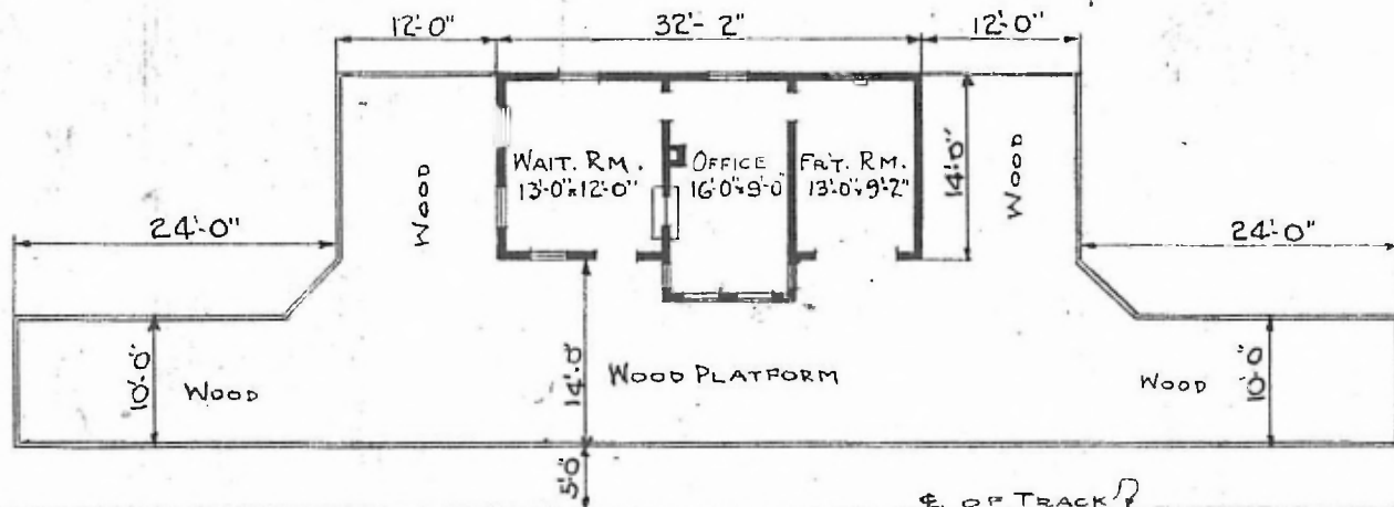
FLOOR PLAN SCALE: \frac{1}{16}'' = 1'-0''
