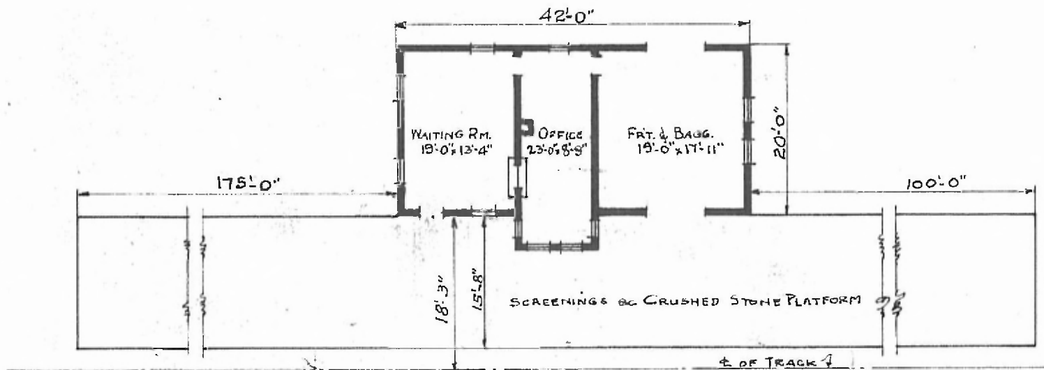
FLOOR PLAN SCALE: \frac{1}{16}'' = 1'-0''
