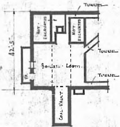
- BOILER ROOM - DIV. CENTRAL SCALE: \frac{1}{32}'' = 1'-0'' SUB-DIV. ARDMORE STA. NO. 559
